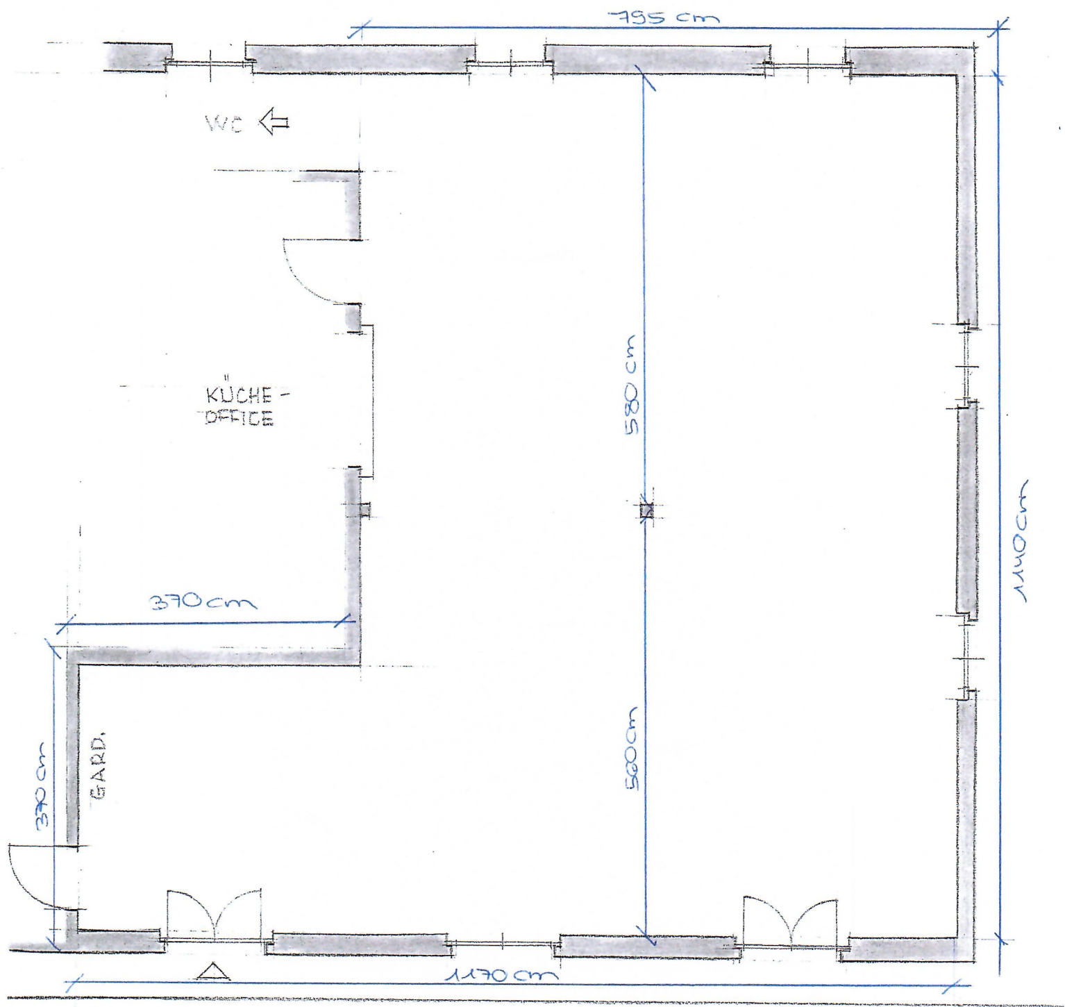
GRUNDRISS SAAL
